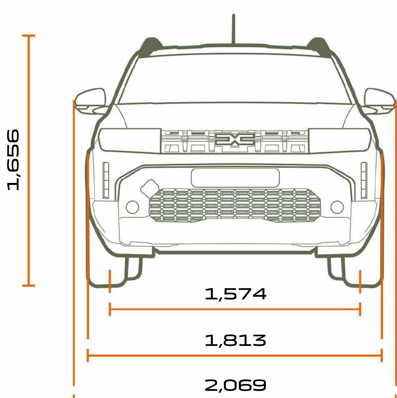
מבט קדמי
