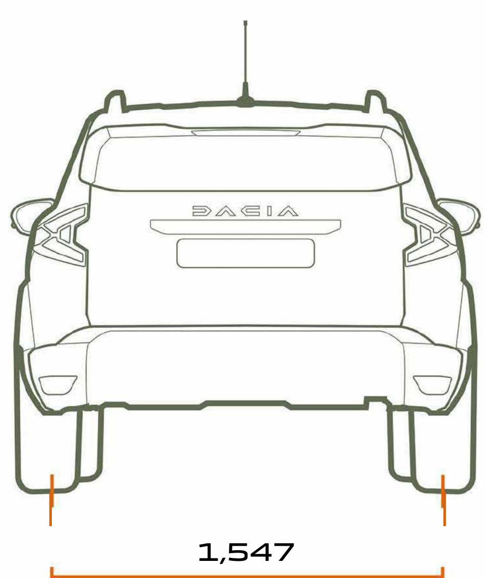
מבט אחורי
