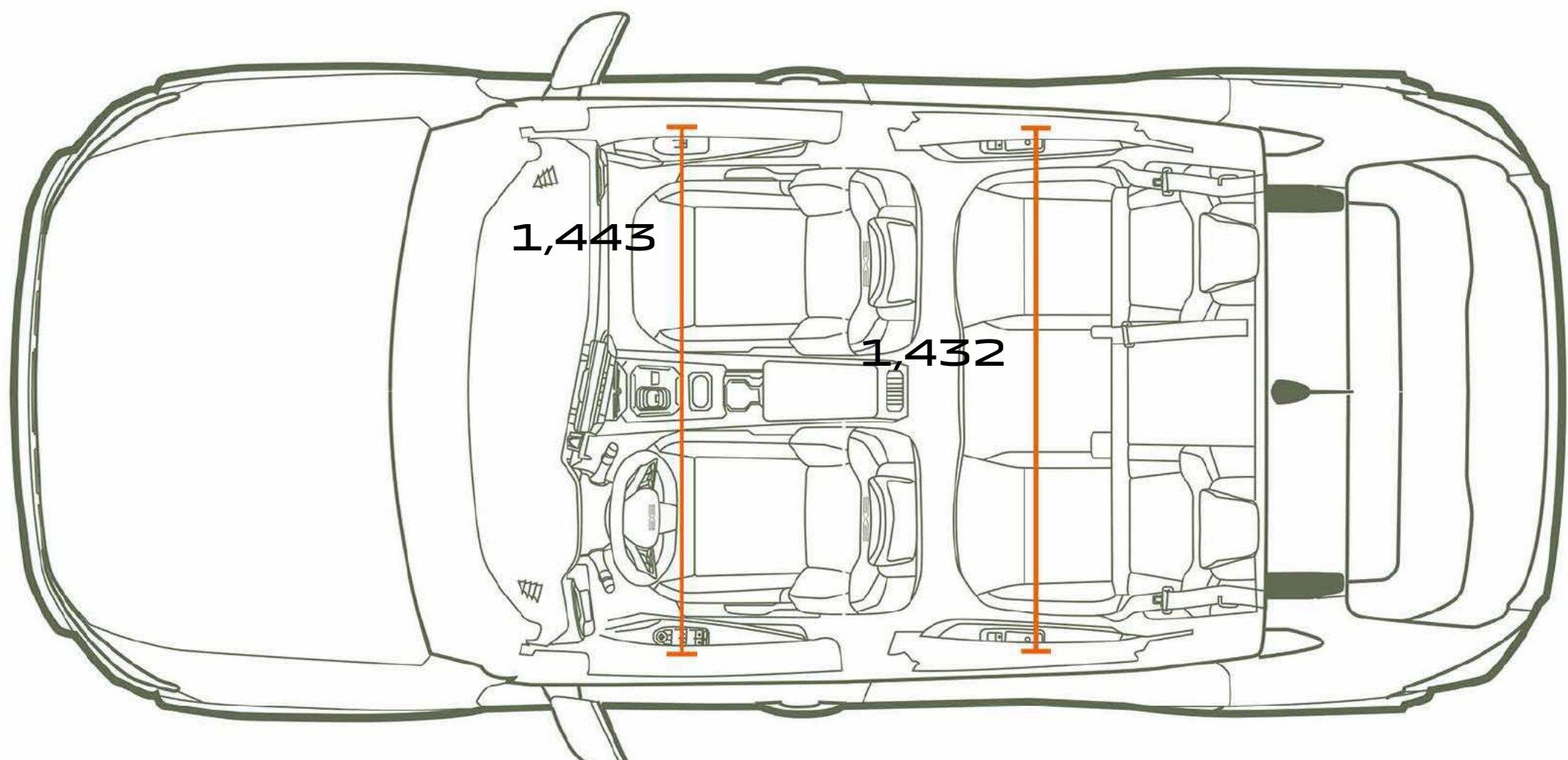
מבט עילי
