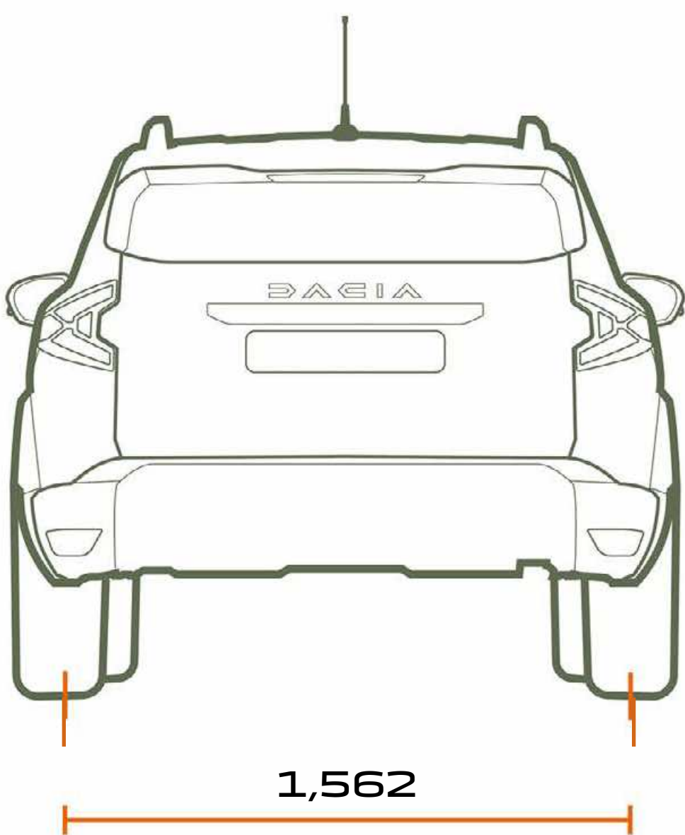
מבט אחורי
