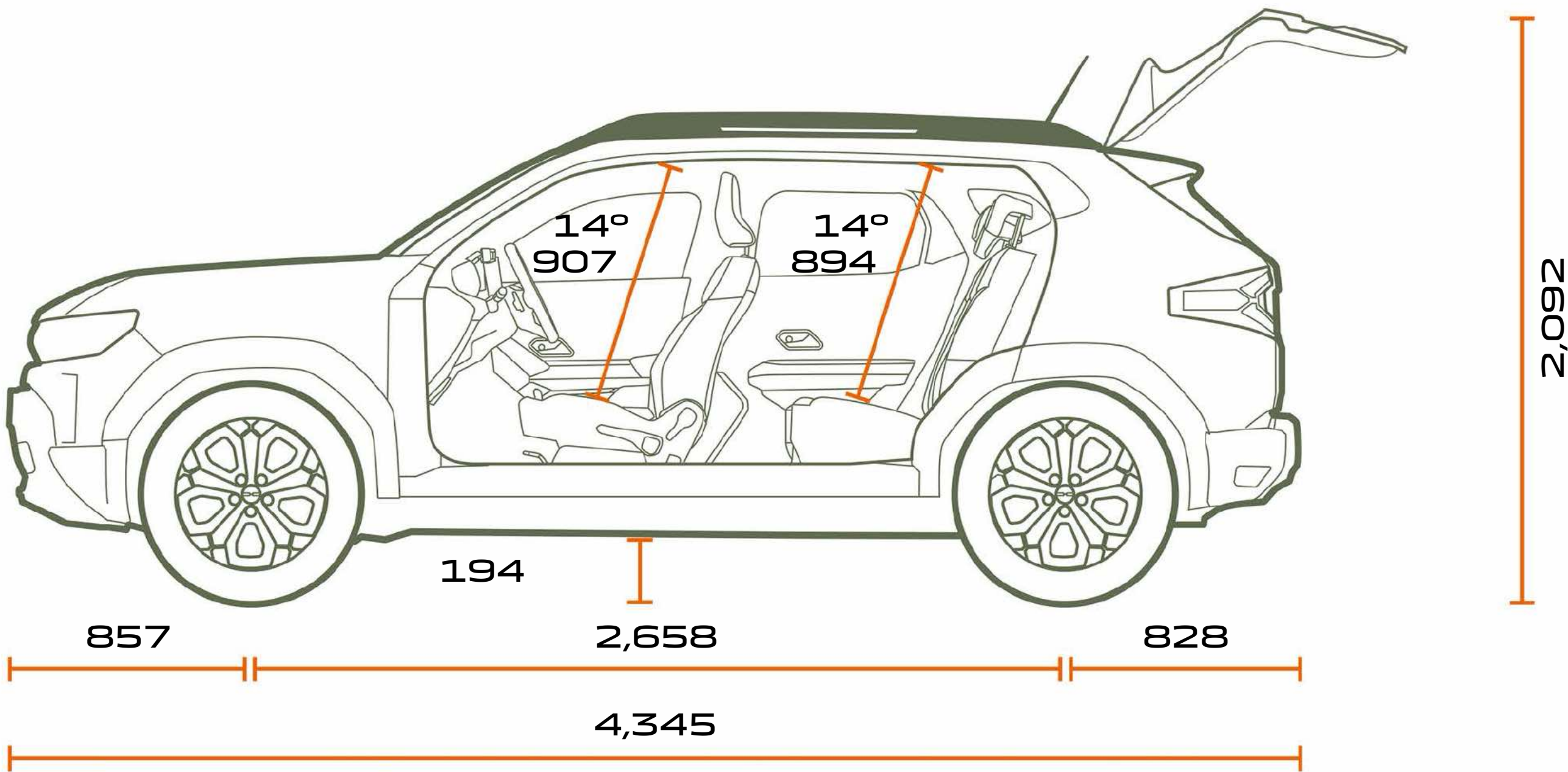
מבט צידי
