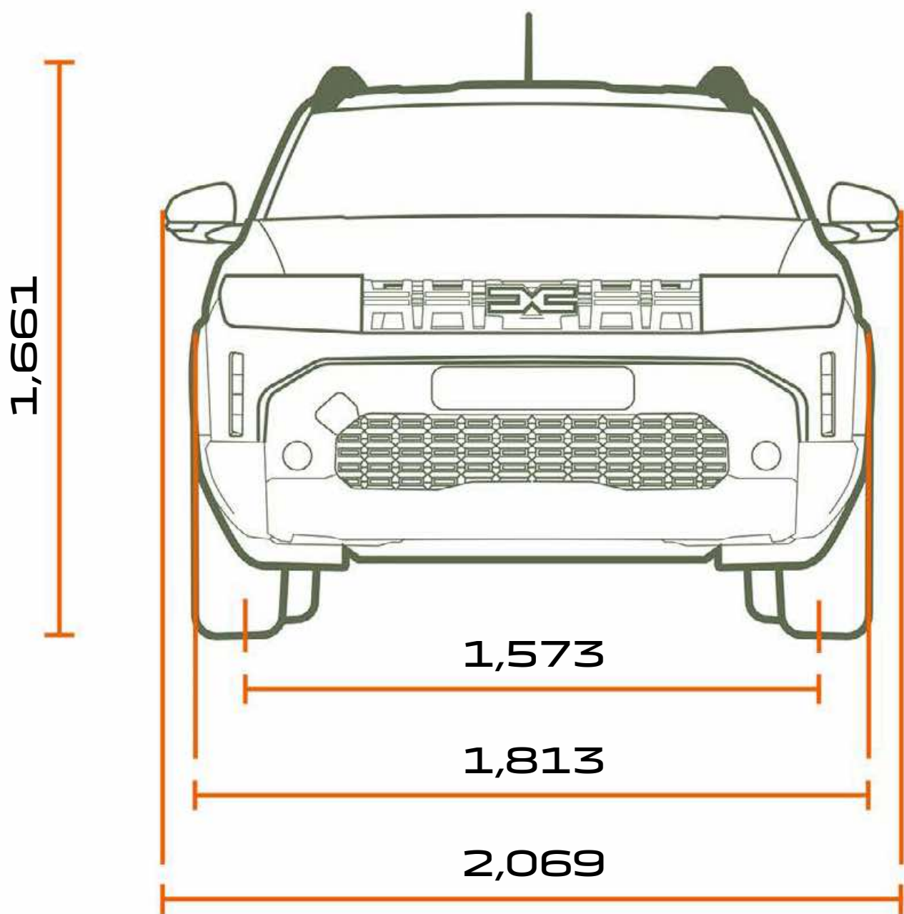
מבט קדמי
