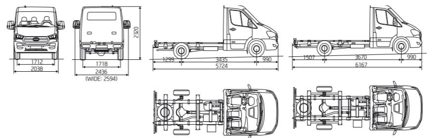
בסיס גלגלים ארוך
