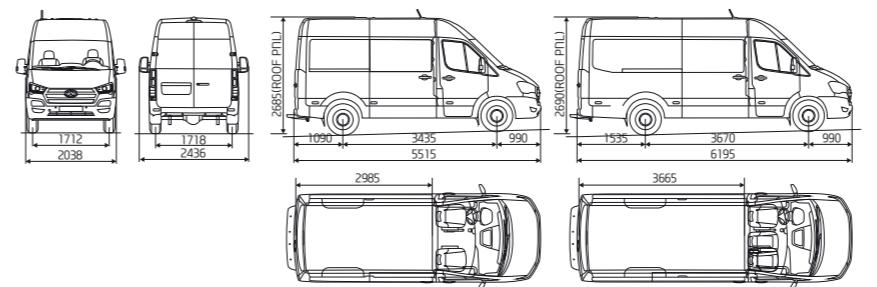
בסיס גלגלים ארוך
